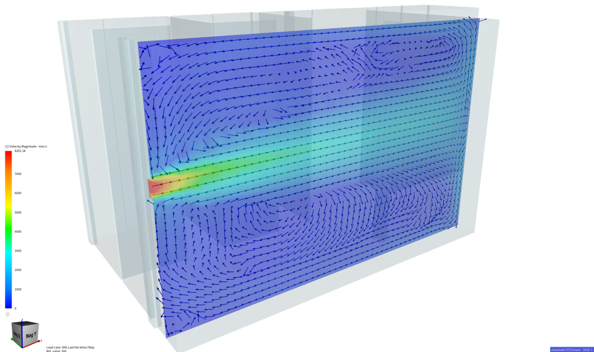
Figura 1: Campo de magnitud de velocidad en el plano vertical longitudinal (vista –Y). Simulación CFD (Autodesk CFD 2020); escala 0–8201 mm/s ( \approx 8,2 \text{ m/s} en el máximo), consistente con la velocidad de impulsión de diseño. Se aprecia la inyección lateral y la recirculación en las zonas periféricas del recinto.
